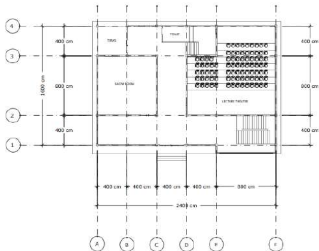
RENCANA DENAH LANTAI 1 SKALA 1 : 200
